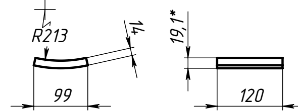
Поз.5 (Упор)
