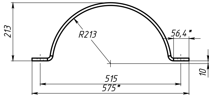
Поз.4 (Полухомут)
