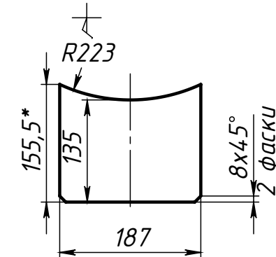
Поз.3 (Ребро среднее)
