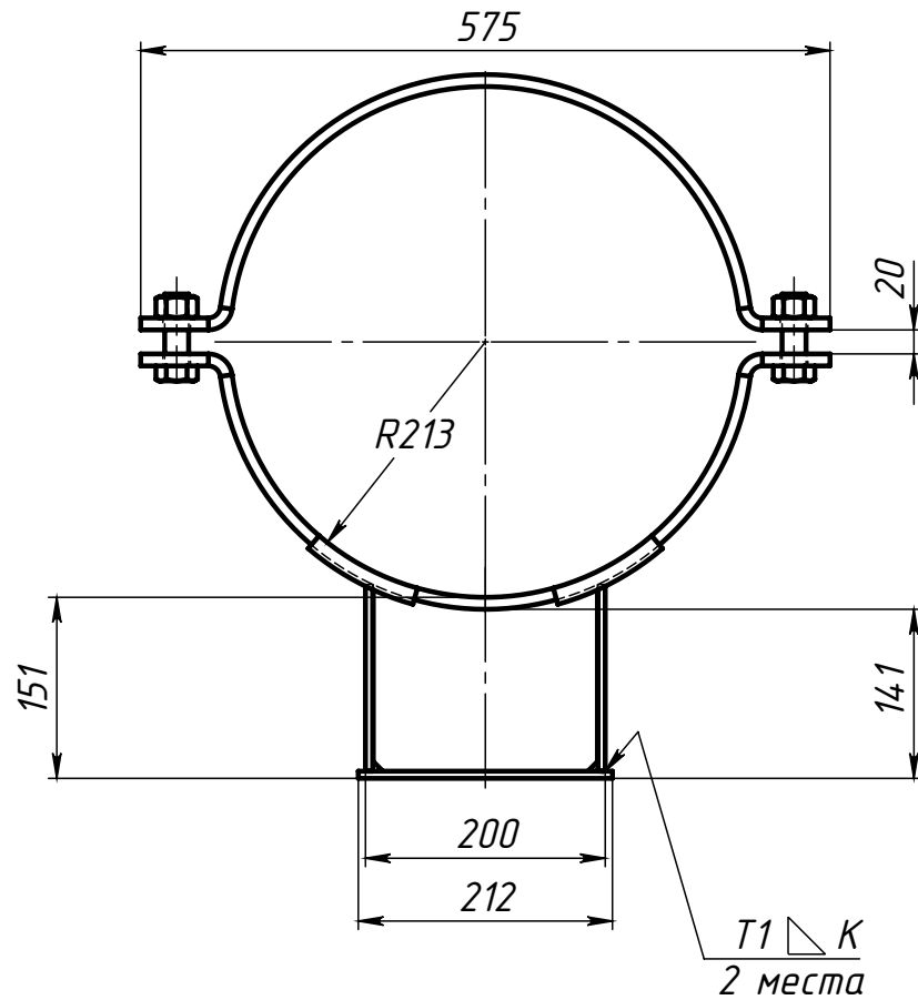
Поз.4 (Полухомут)
